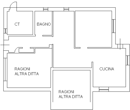
PIANO TERRA H=3.00
